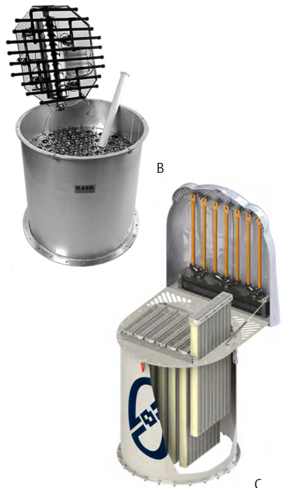
Bild 15: Silo Be- und Entlüftungsfilter als Spülluftfilter ausgeführt (A, B: Schlauchfilter, C: Taschenfilter) (A, B: AZO GmbH + Co. KG, C: WAM GmbH)
